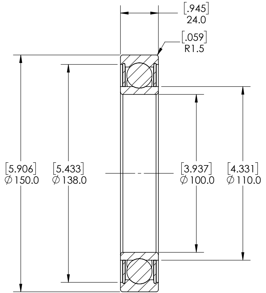
SECTION A-A
